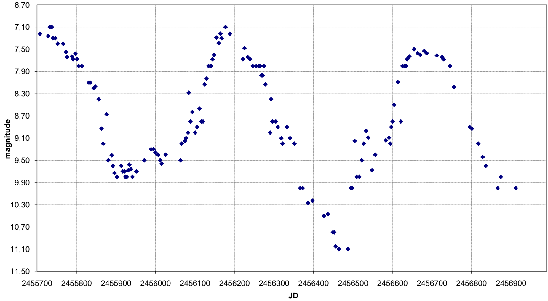
U Cyg - Grafico al 11/09/2014
