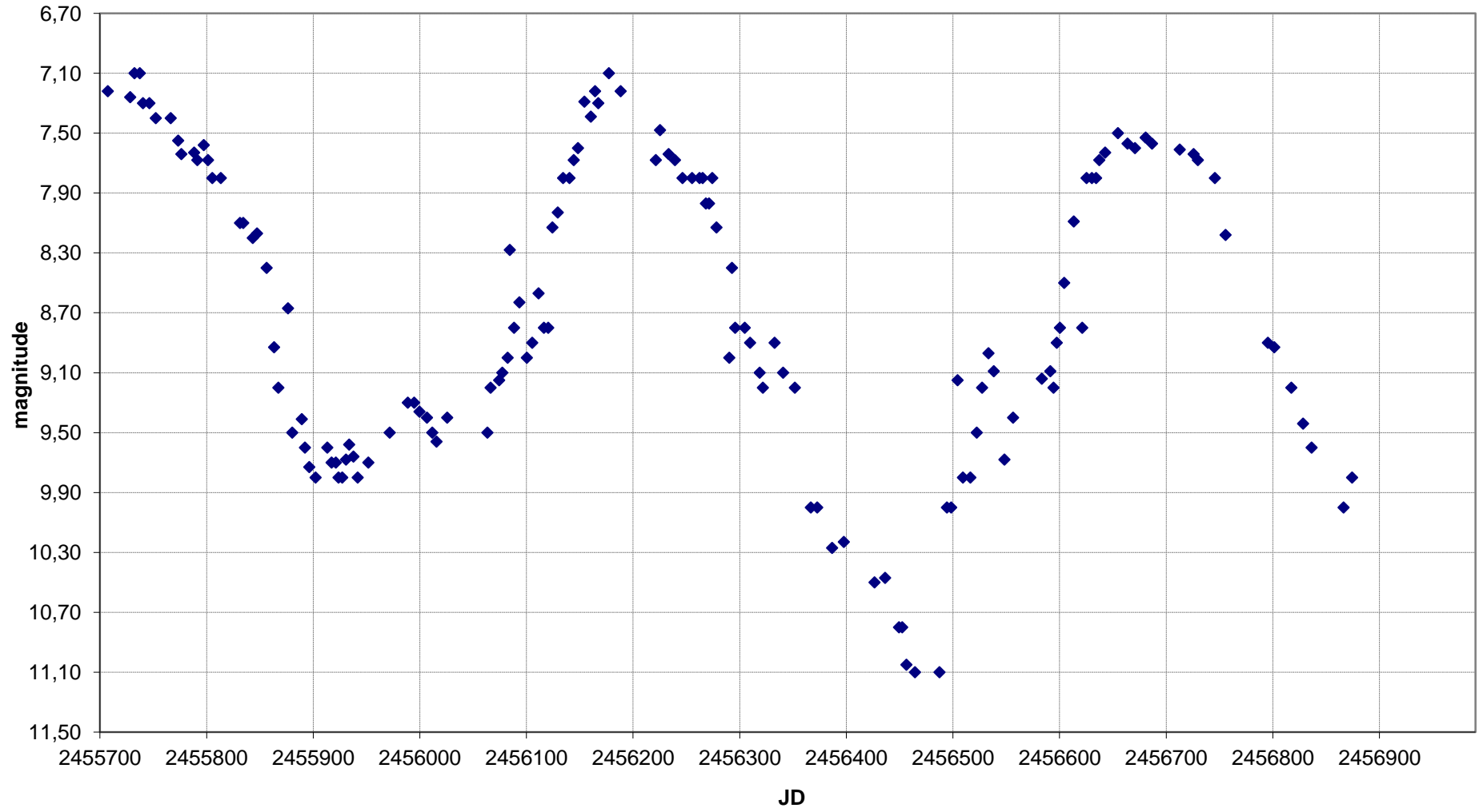
U Cyg - Grafico al 04/08/2014
