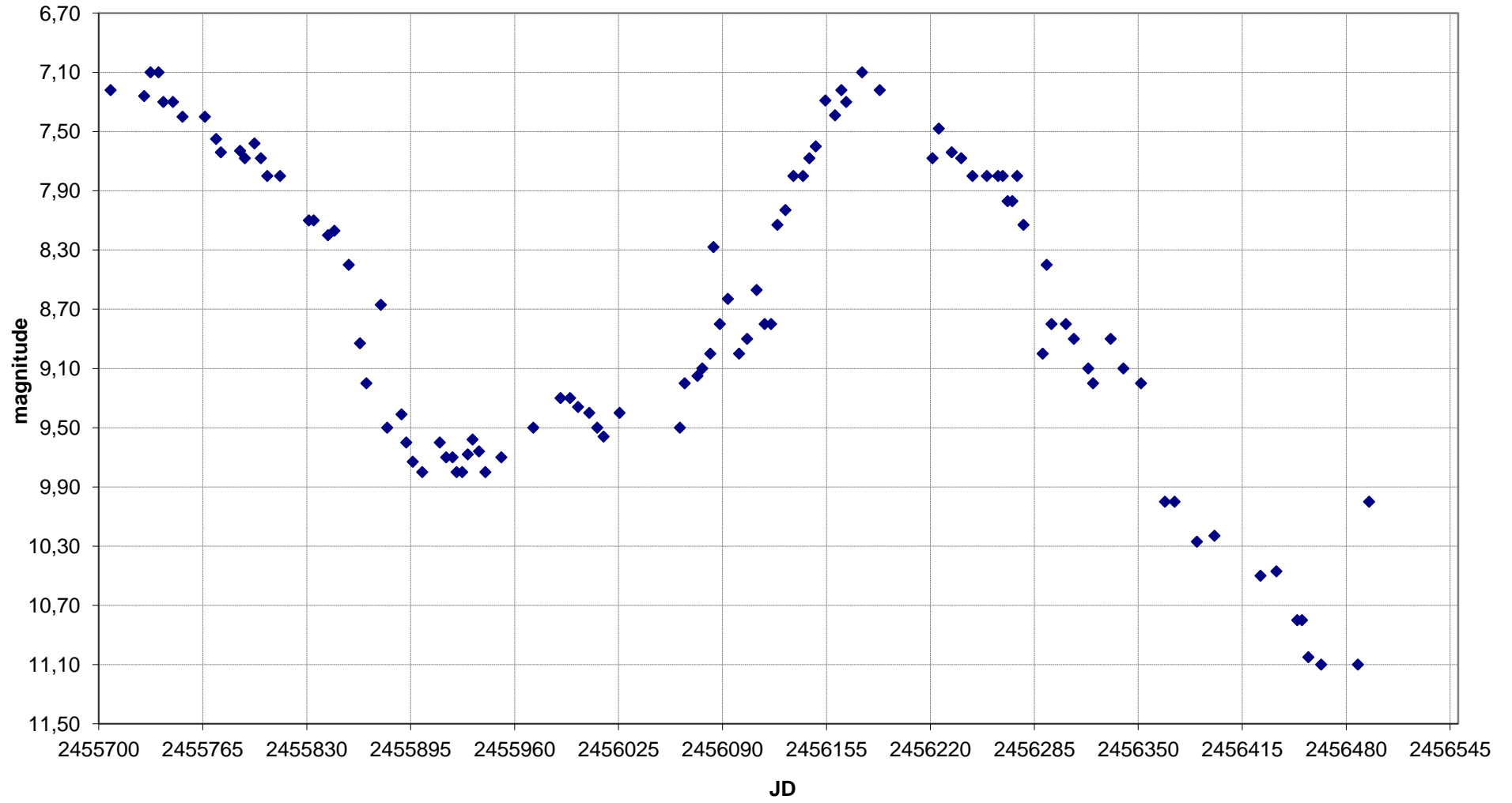
U Cyg - Grafico al 20/07/2013
