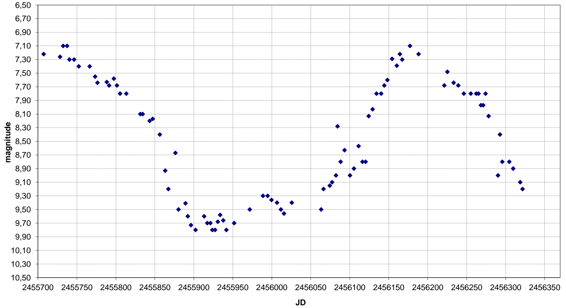
U Cyg - Grafico al 29/01/2013
