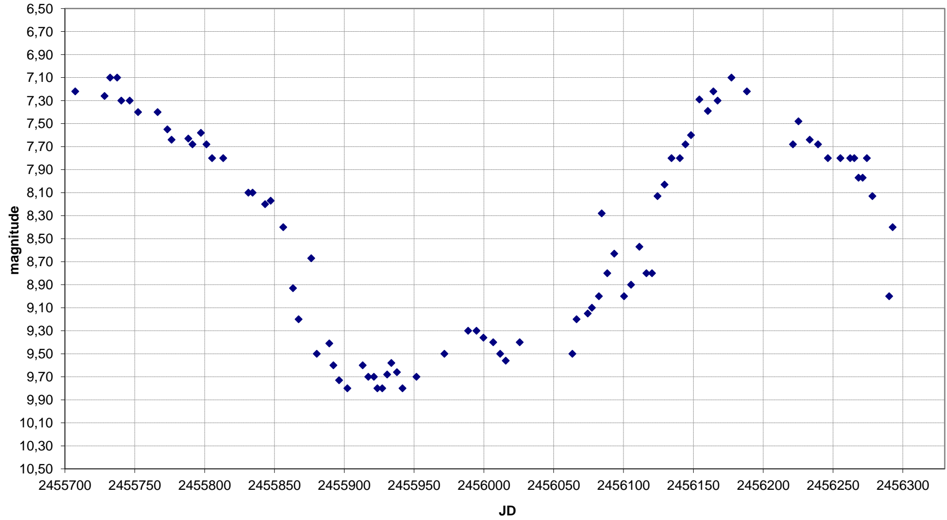
U Cyg - Grafico al 31/12/2012
