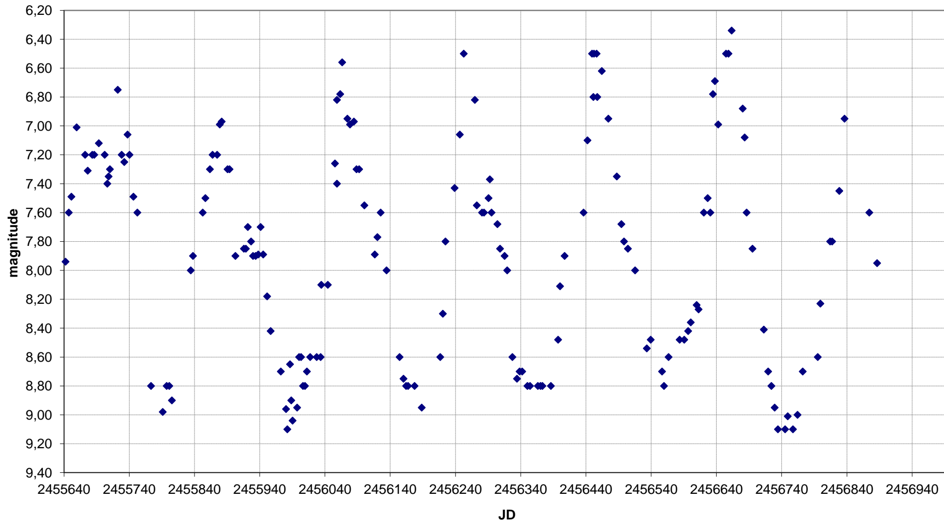
Z UMa - Grafico al 16/08/2014
