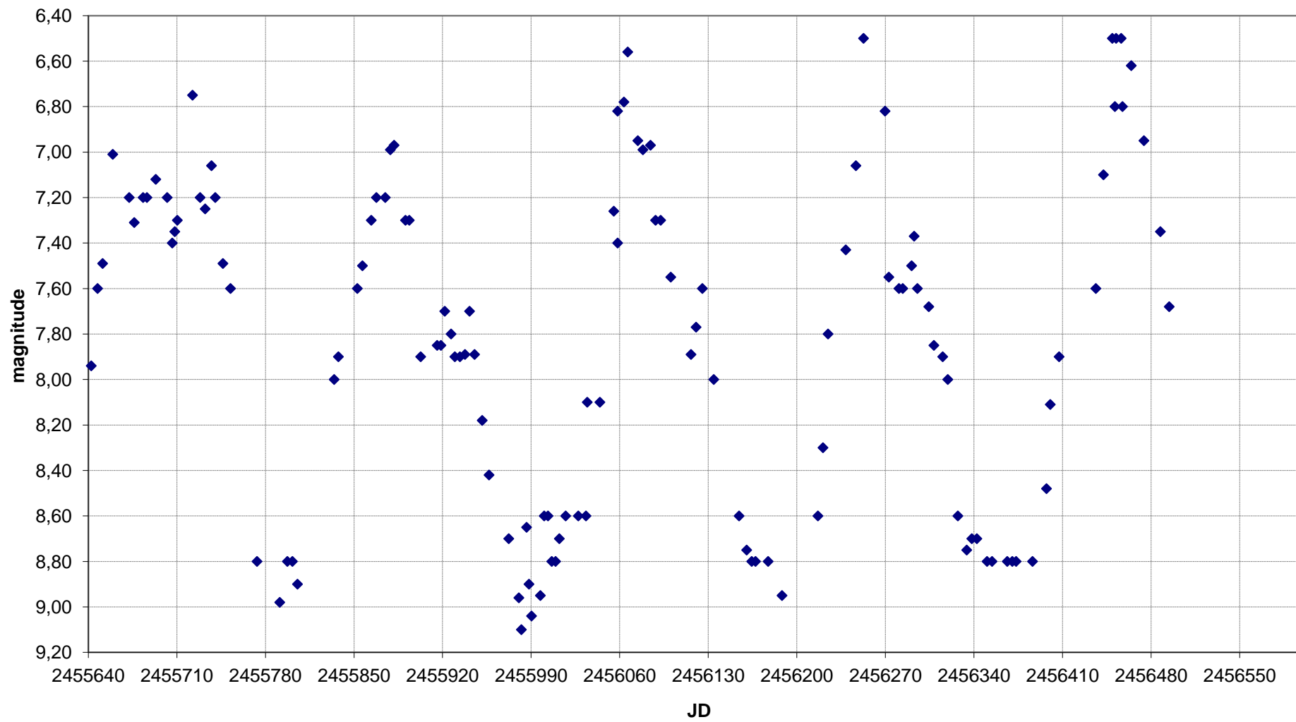
Z UMa - Grafico al 20/07/2013
