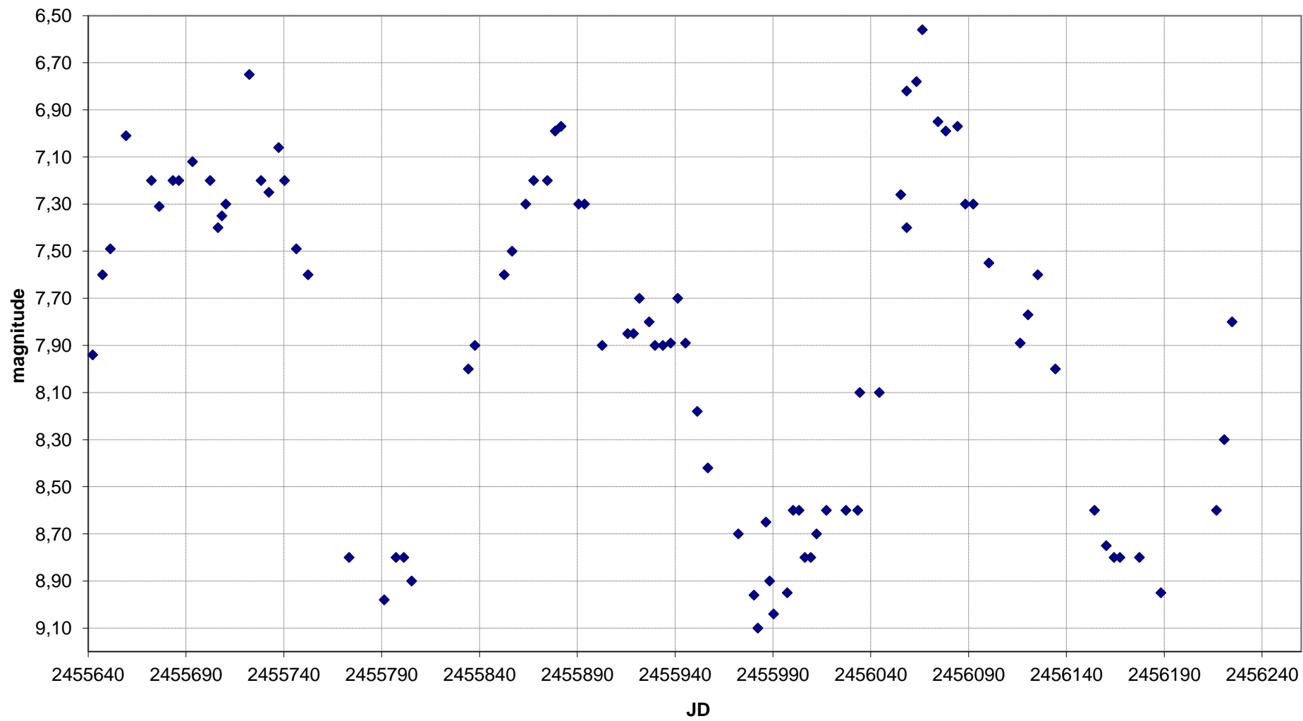
Z UMa - Grafico al 24/10/2012
