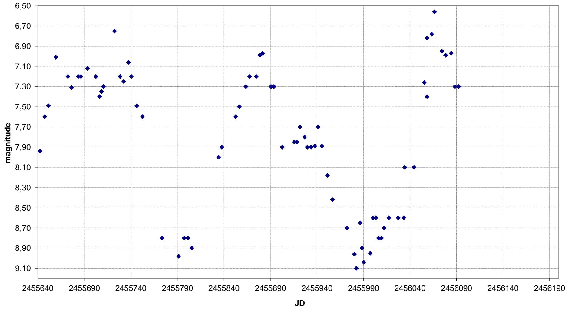
Z UMa - Grafico al 13/06/2012
