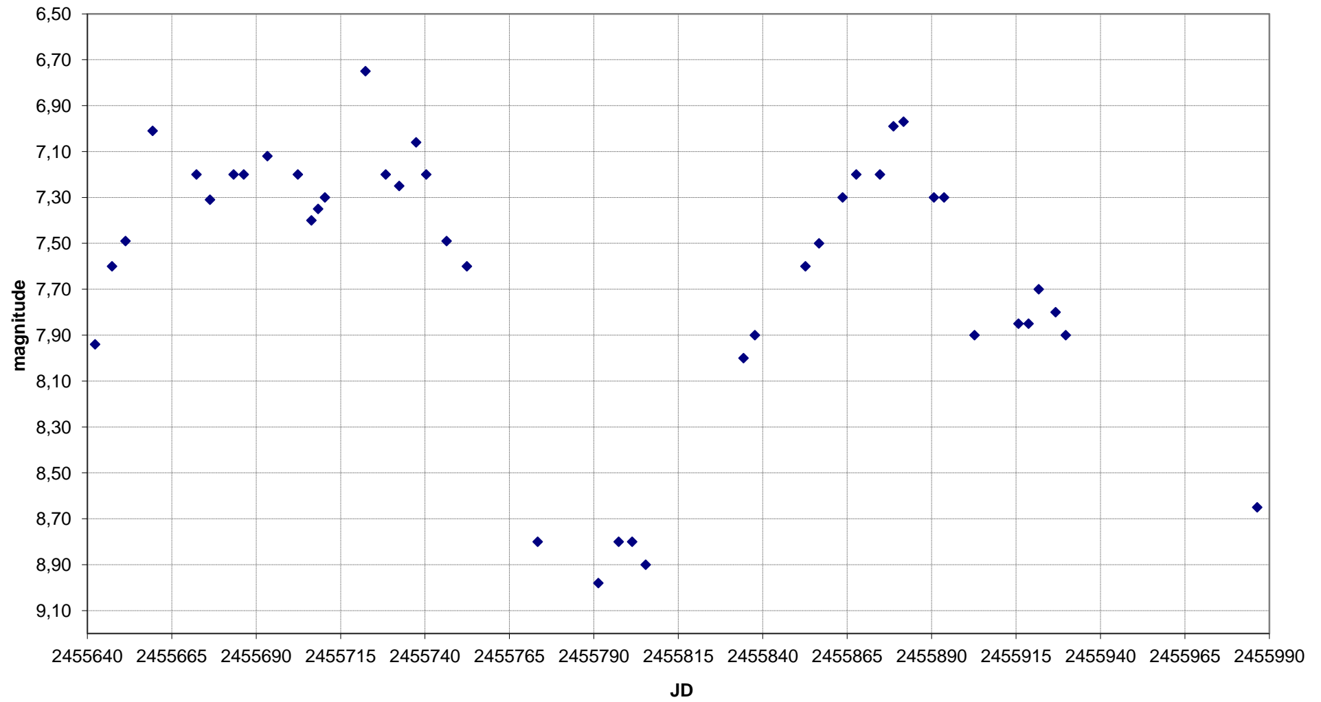
Z UMa - Grafico al 28/02/2012
