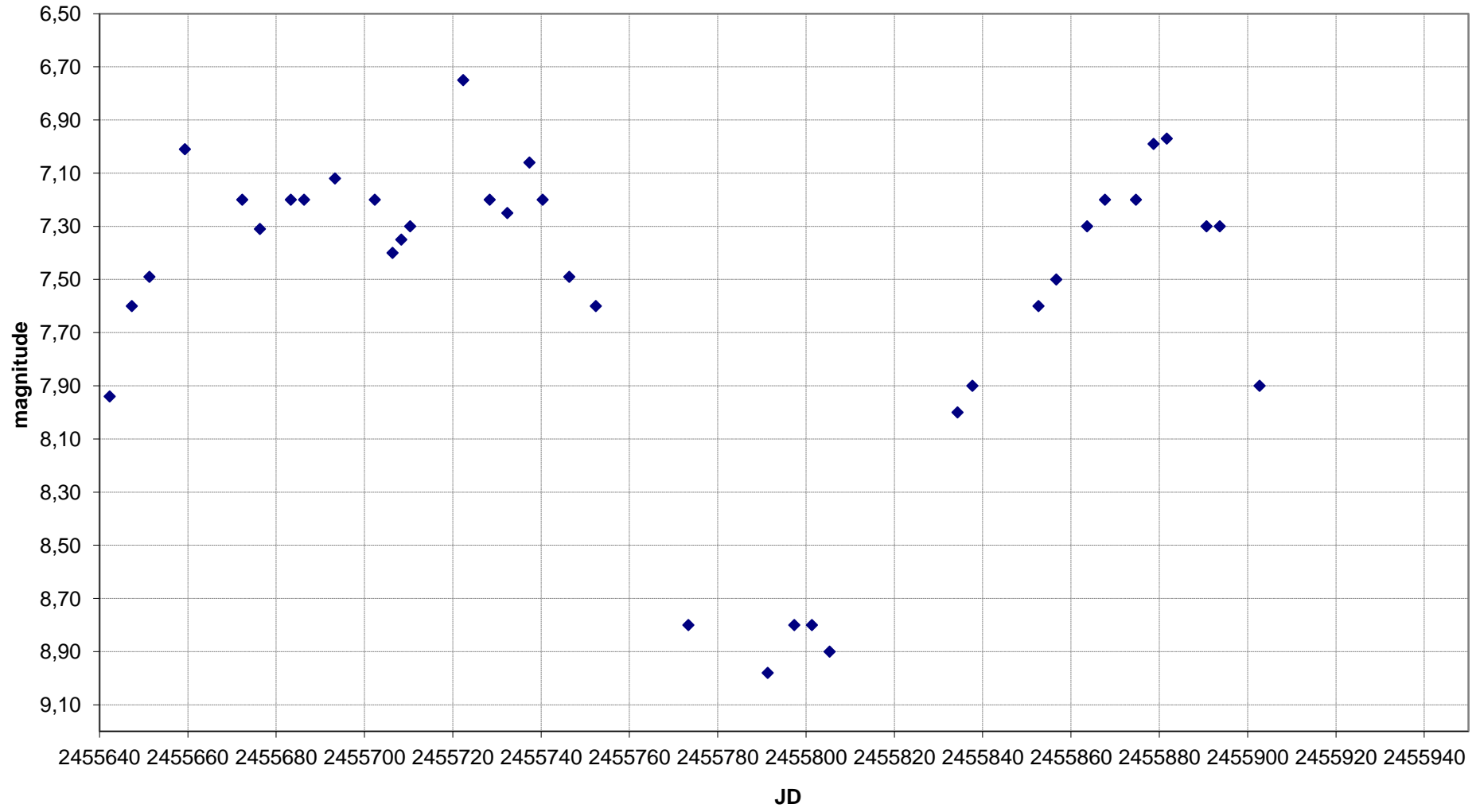
Z UMa - Grafico al 07/12/2011
