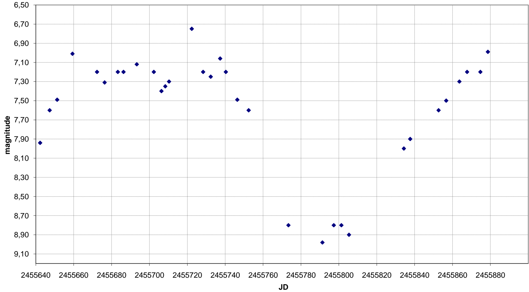
Z UMa - Grafico al 13/11/2011
