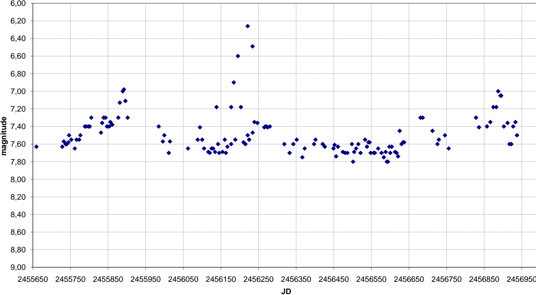
V Aql - Grafico al 06/10/2014
