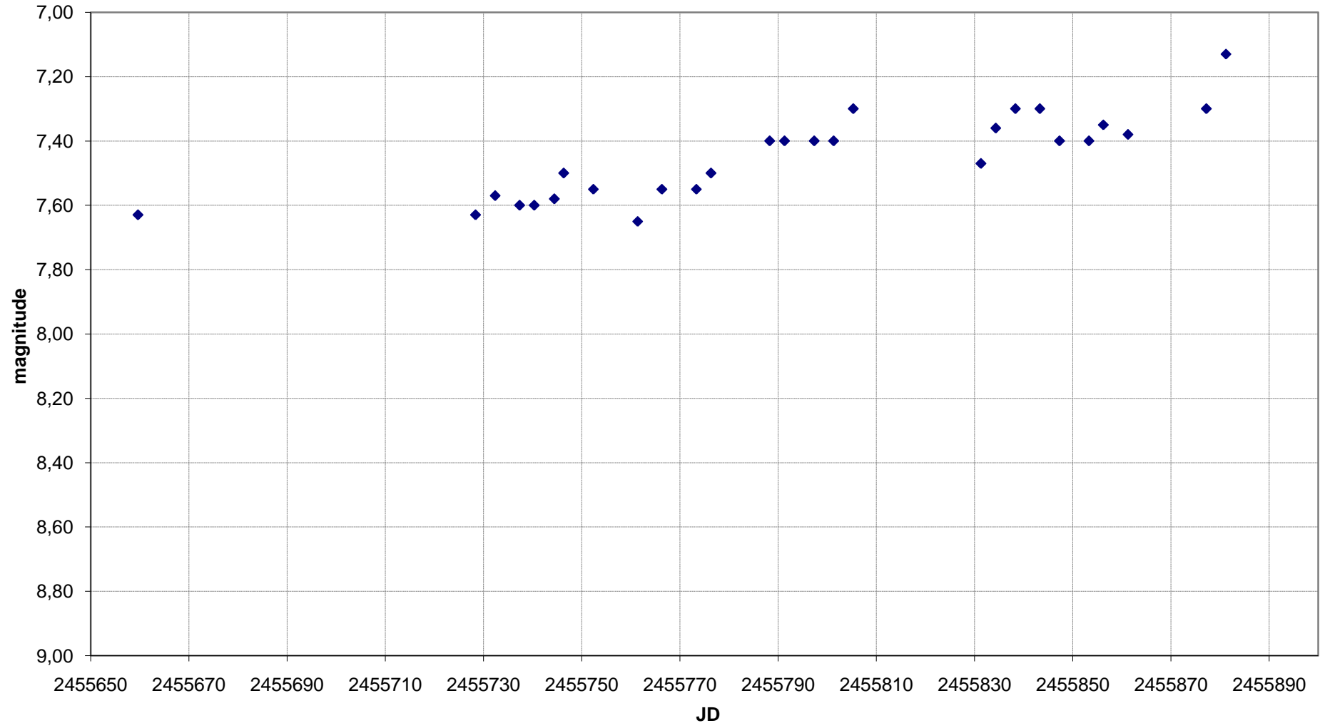
V Aql - Grafico al 15/11/2011
