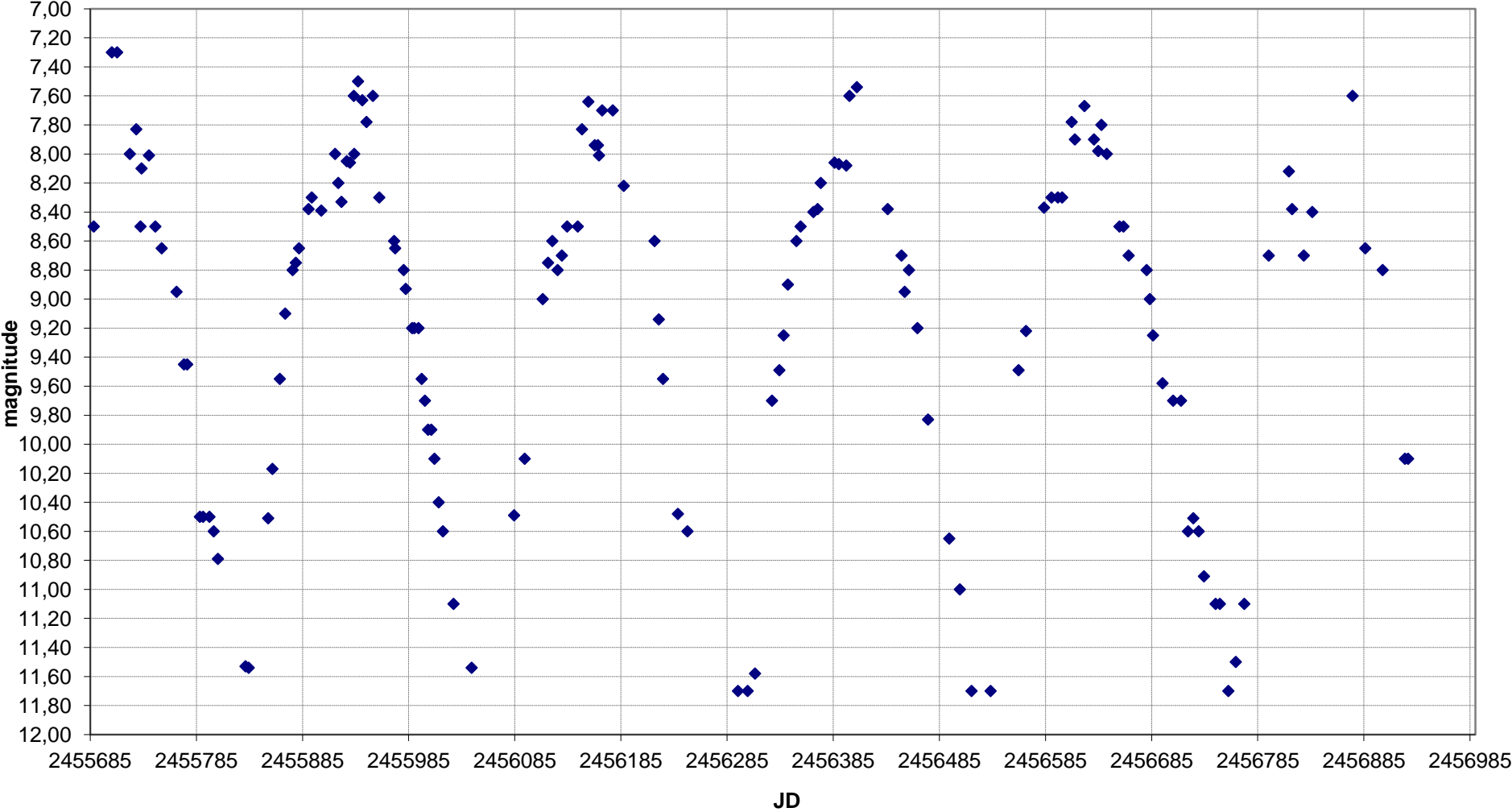
S UMa - Grafico al 26/09/2014
