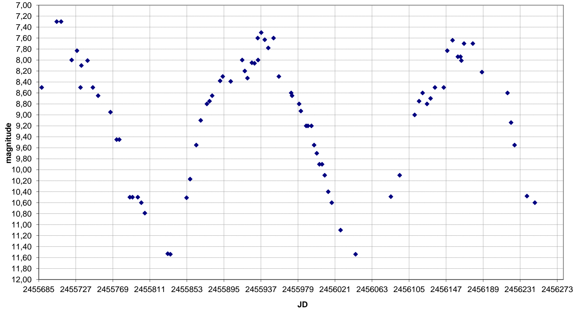
S UMa - Grafico al 16/11/2012
