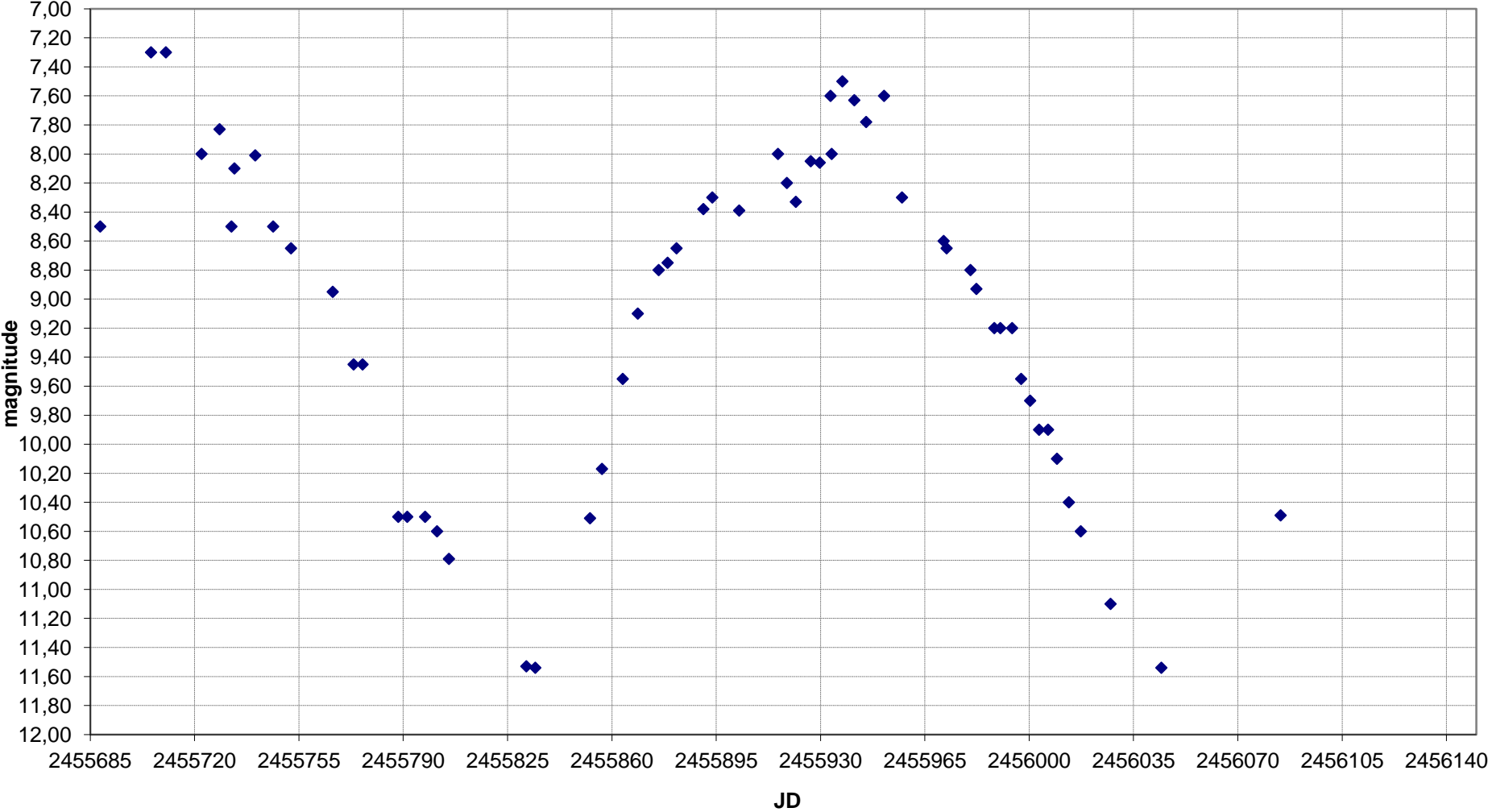
S UMa - Grafico al 05/06/2012
