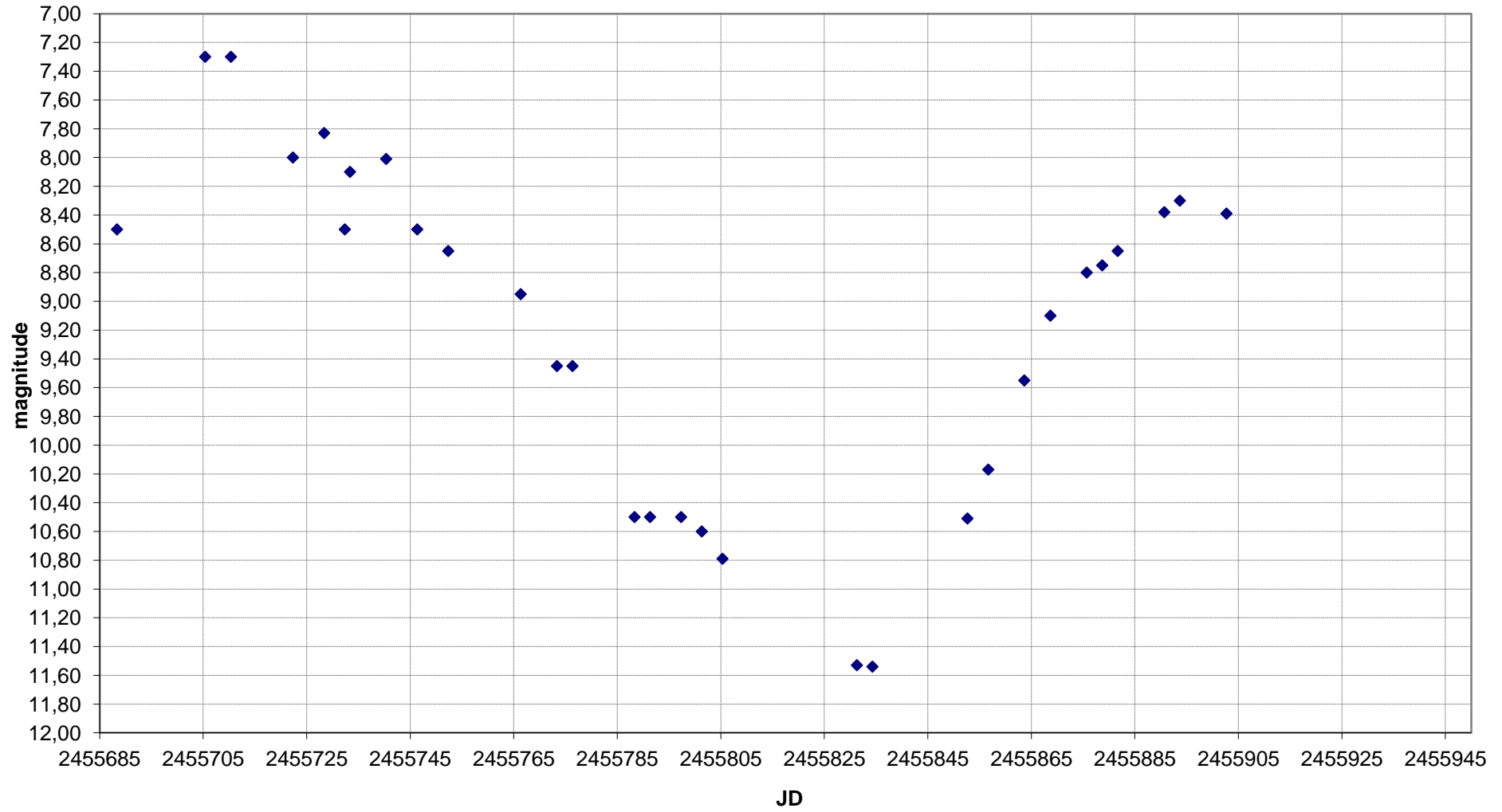
S UMa - Grafico al 07/12/2011
