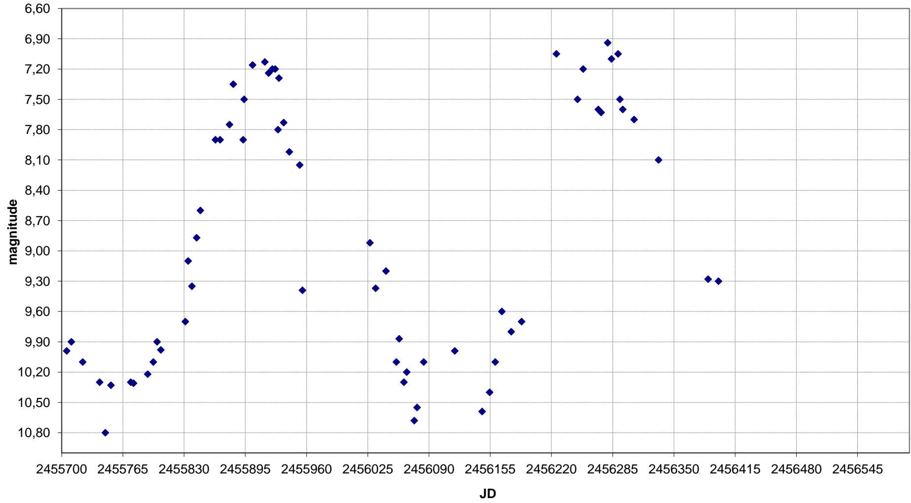
V CrB - Grafico al 14/04/2013
