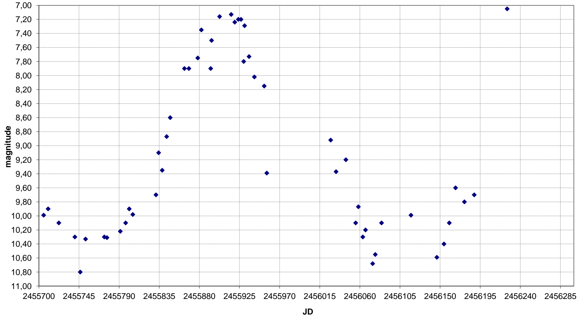
V CrB - Grafico al 24/10/2012
