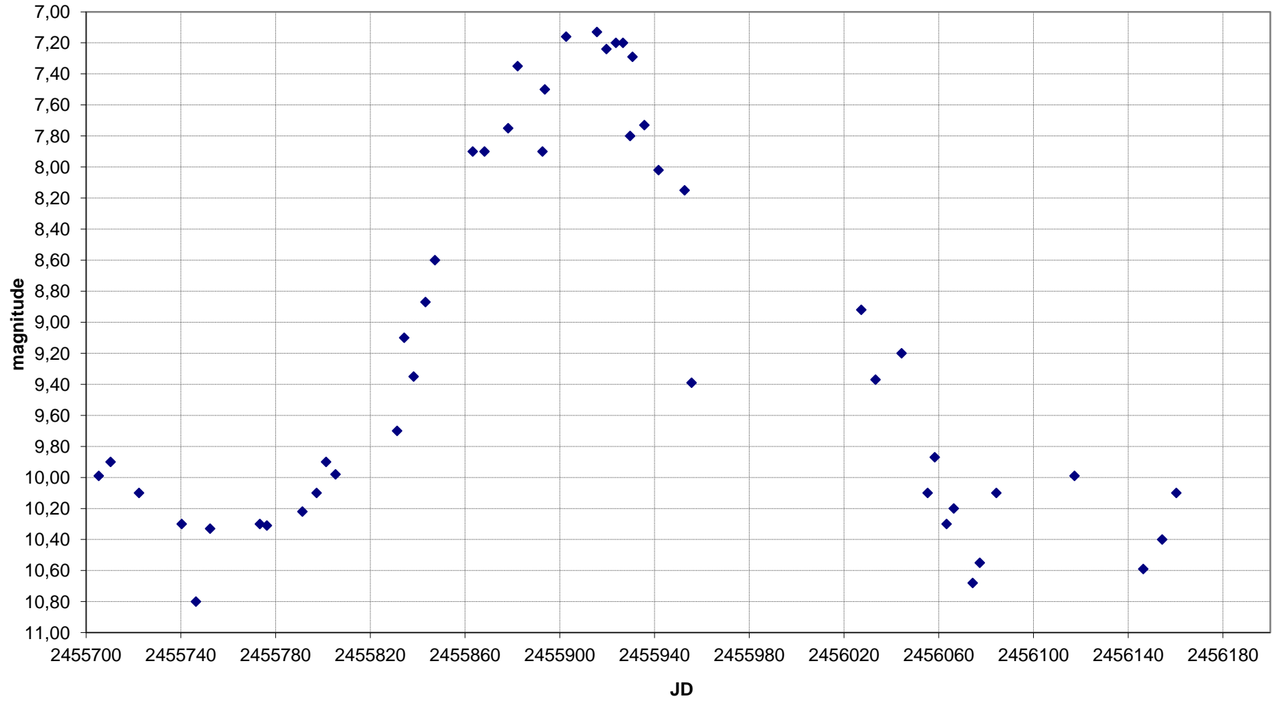
V CrB - Grafico al 20/08/2012
