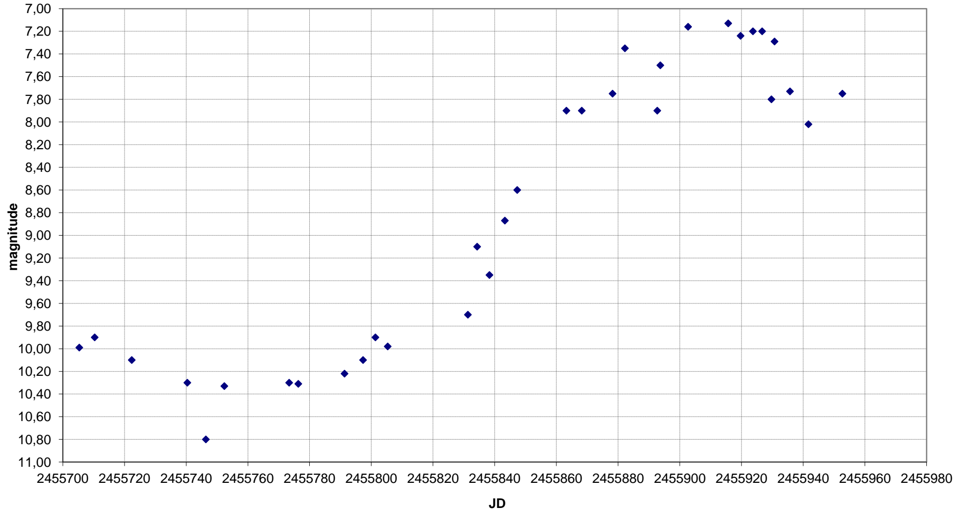
V CrB - Grafico al 26/01/2012
