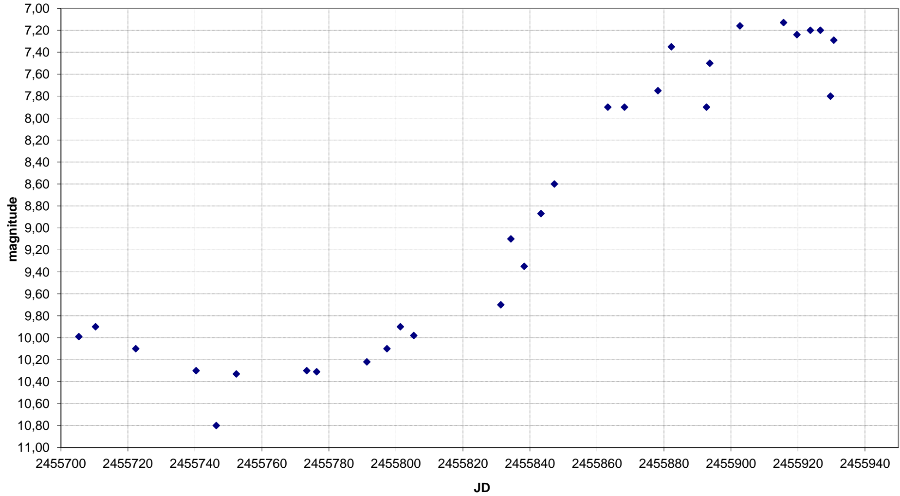
V CrB - Grafico al 04/01/2012
