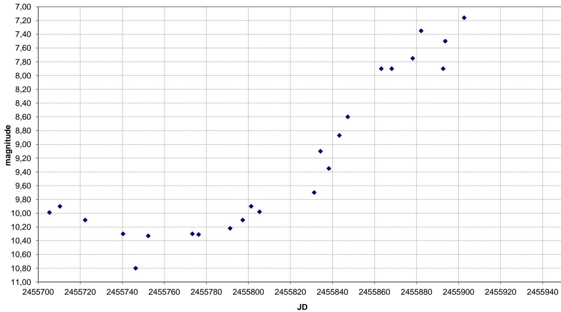
V CrB - Grafico al 07/12/2011
