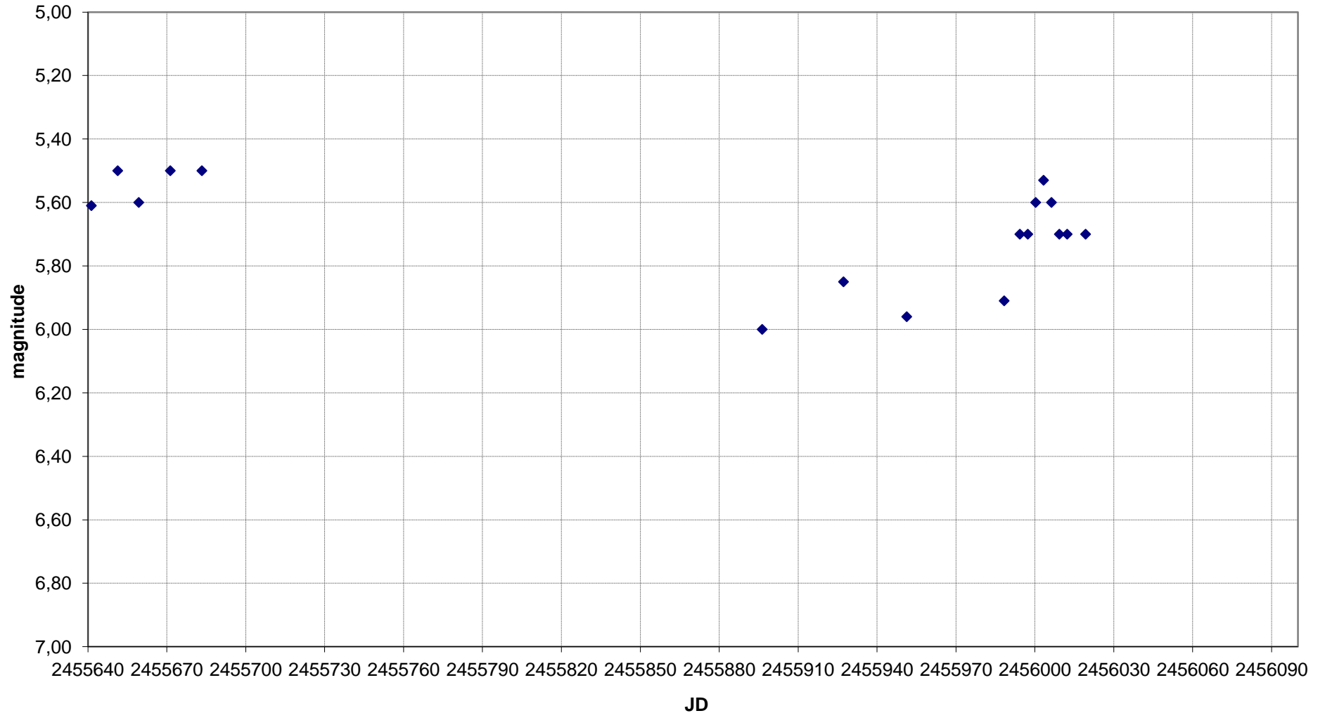
UU Aur - Grafico al 01/04/2012
