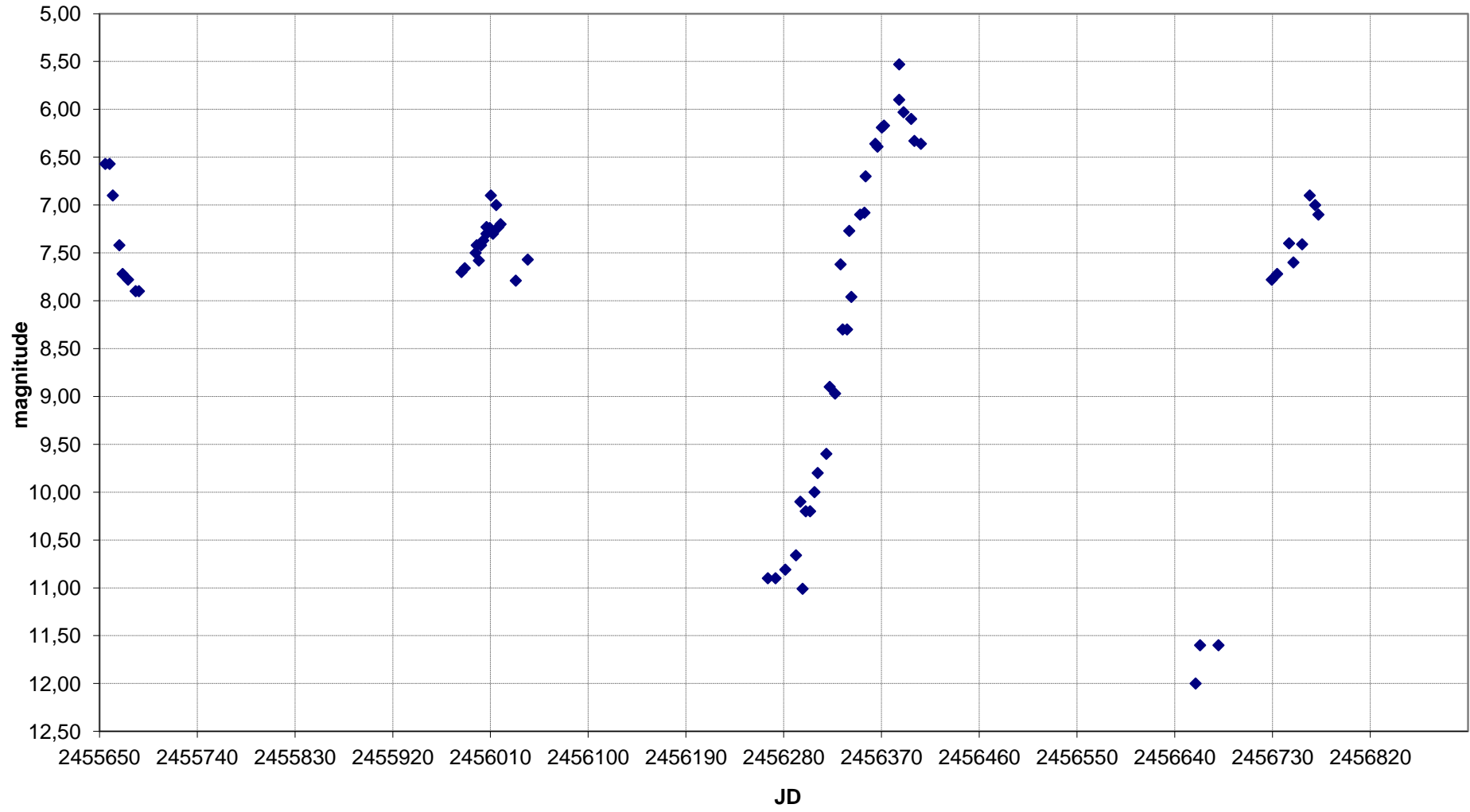
U Ori - Grafico al 24/04/2014
