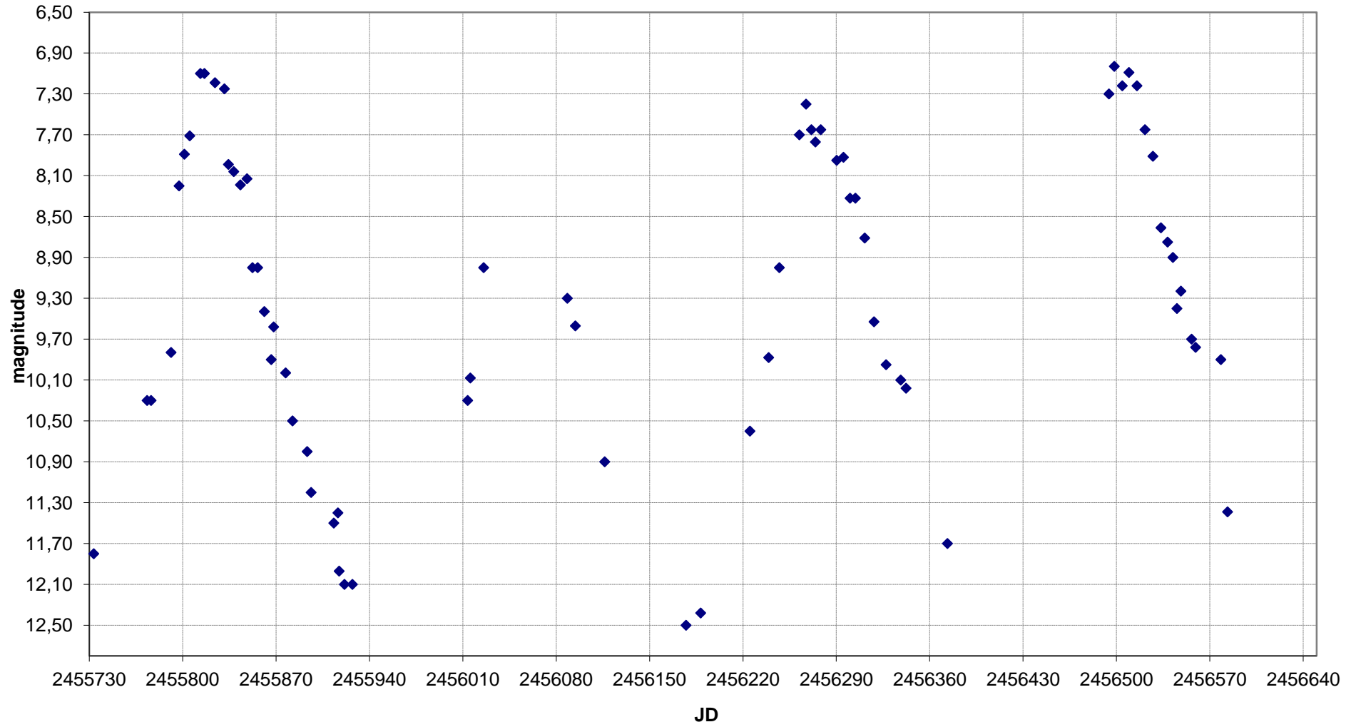
V Cas - Grafico al 17/10/2013
