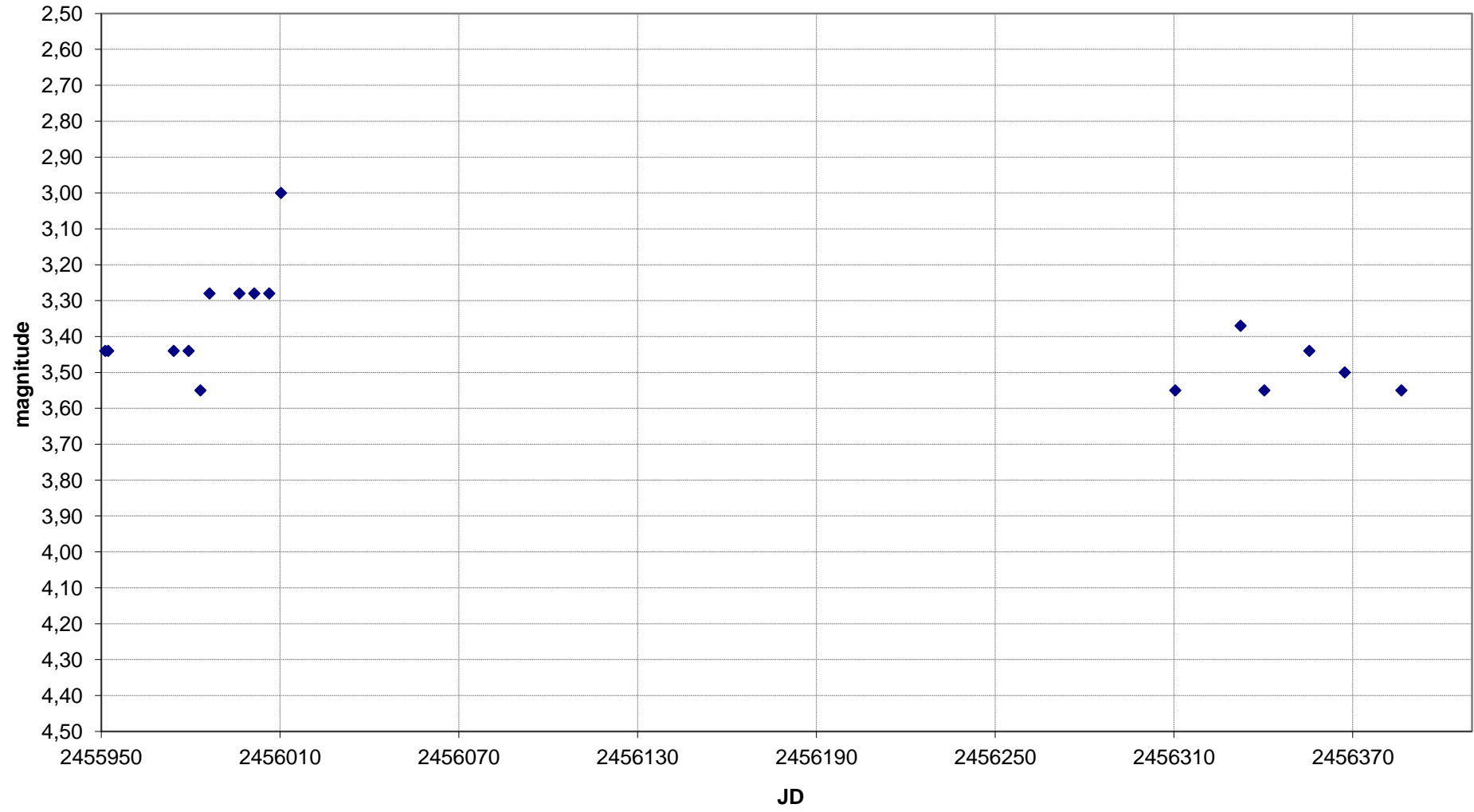
Eta Gem - Grafico al 03/04/2013
