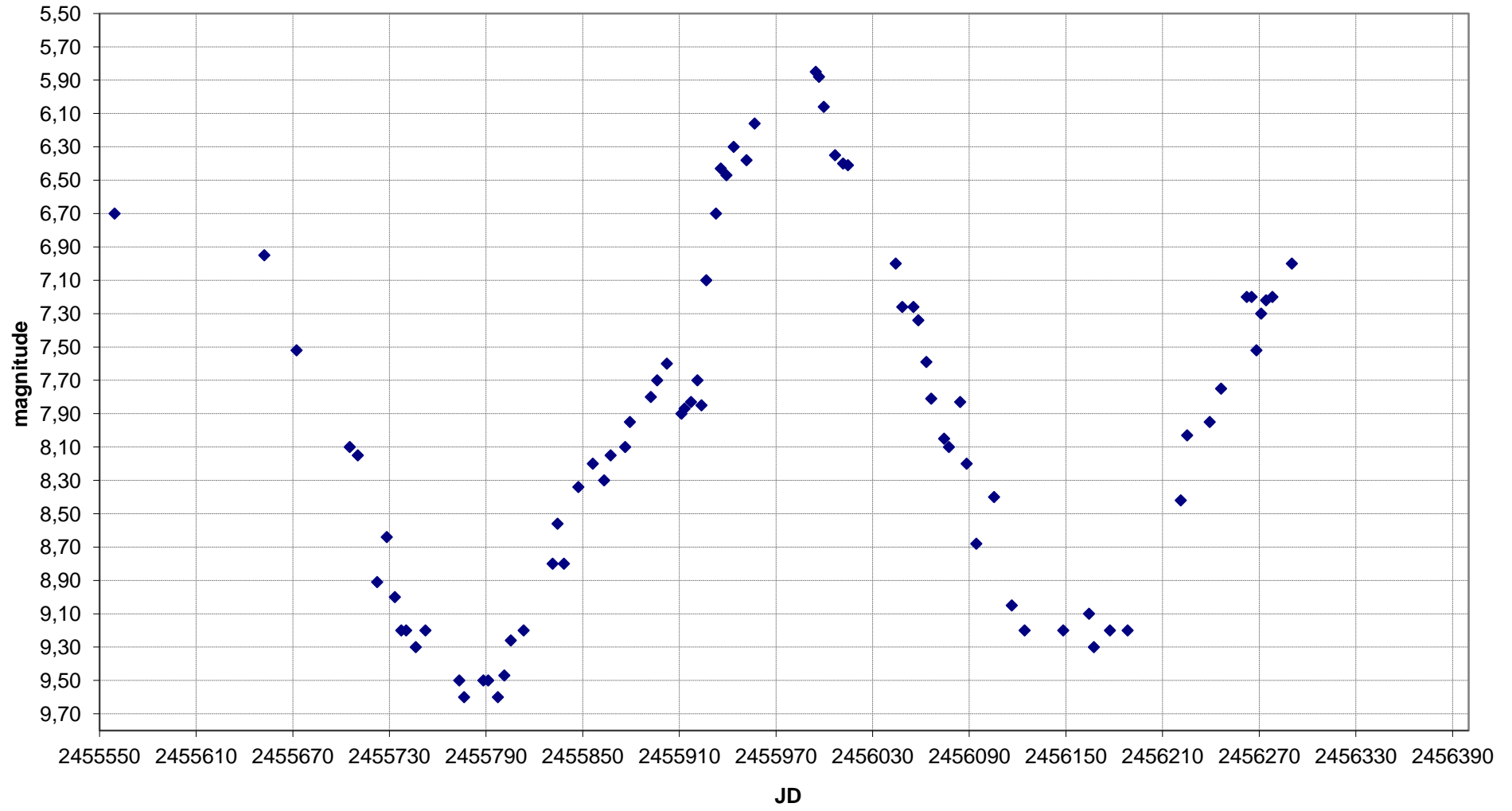
T Cep - Grafico al 28/12/2012
