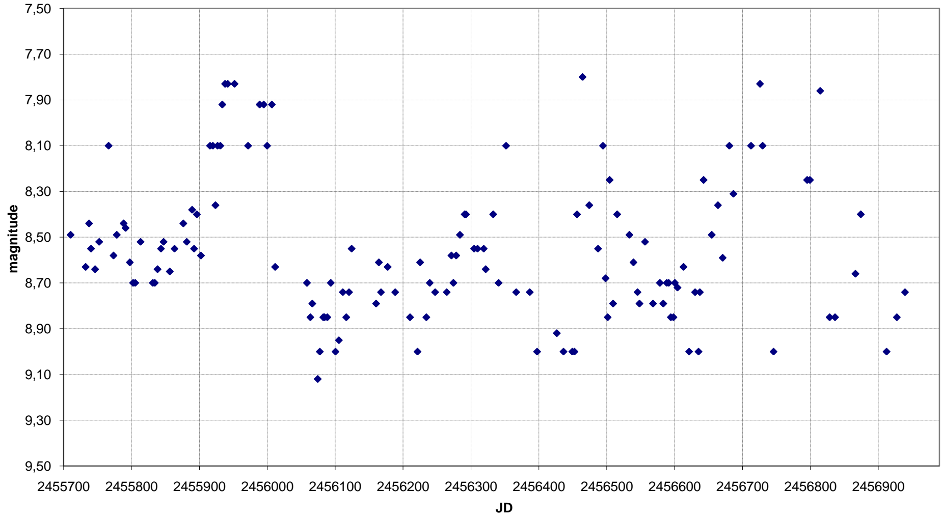
T Lyr - Grafico al 08/10/2014
