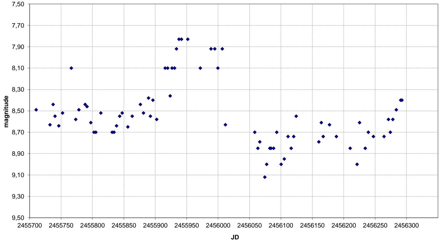
T Lyr - Grafico al 31/12/2012
