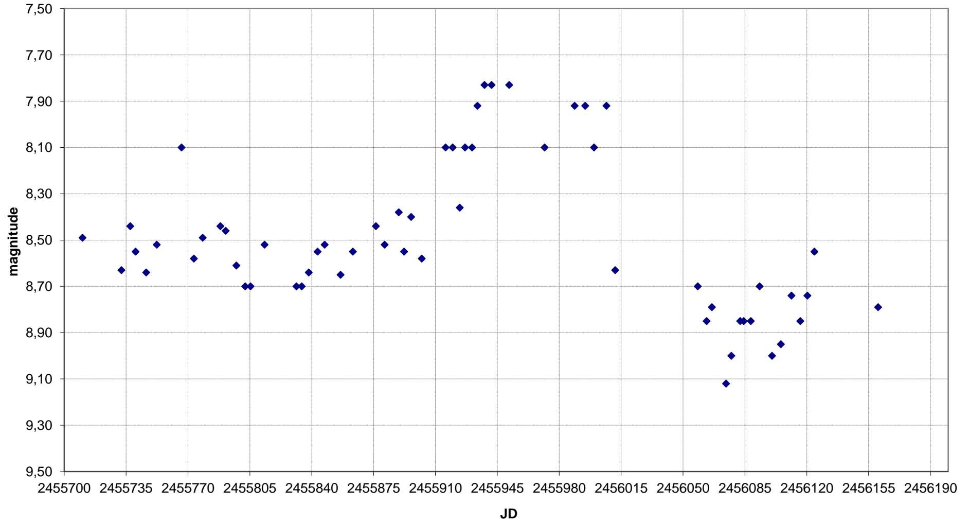
T Lyr - Grafico al 20/08/2012
