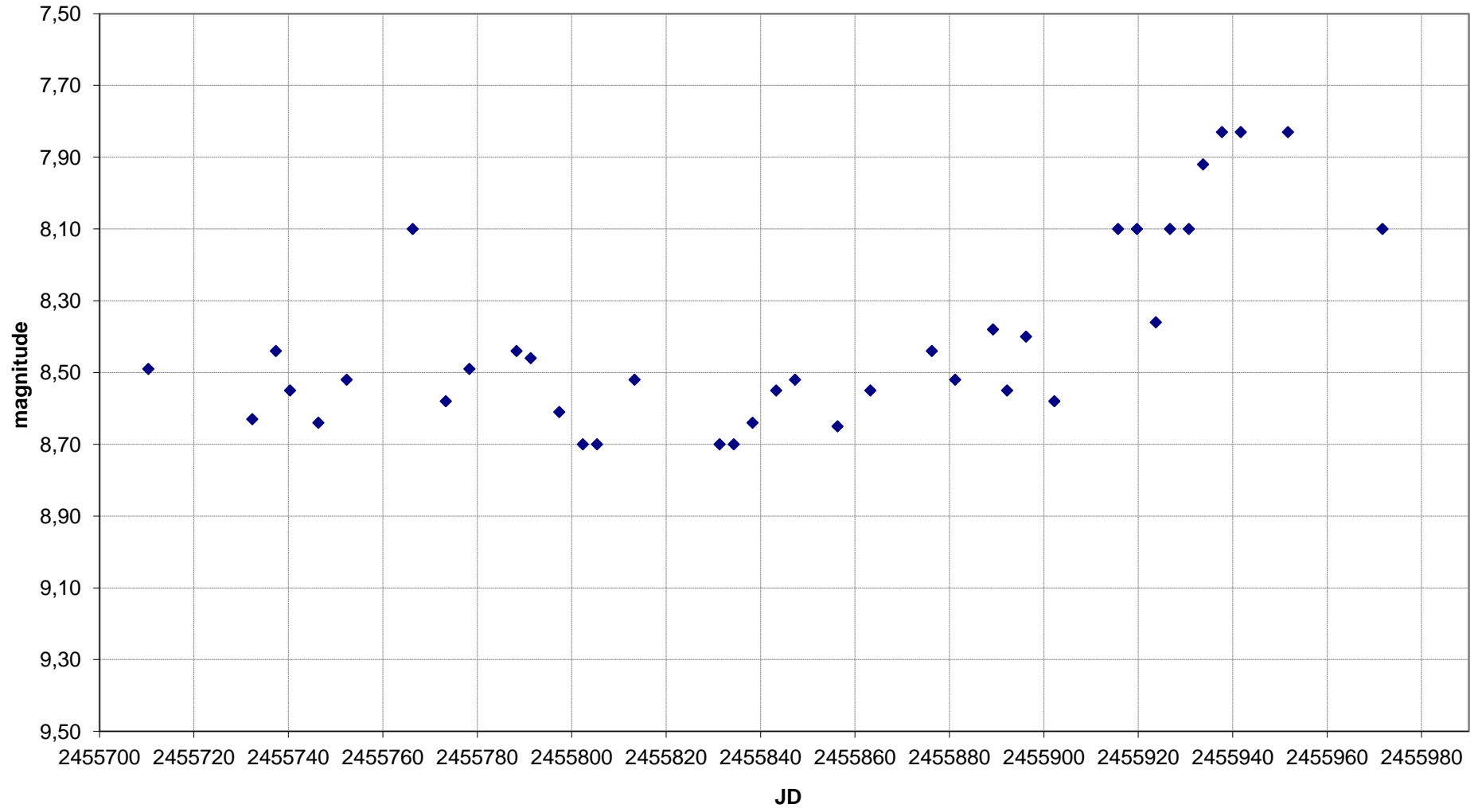
T Lyr - Grafico al 14/02/2012
