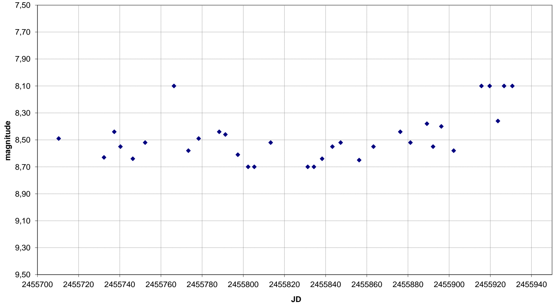
T Lyr - Grafico al 04/01/2012
