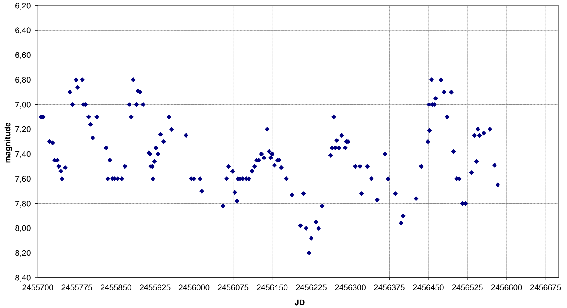
AF Cyg - Grafico al 17/10/2013
