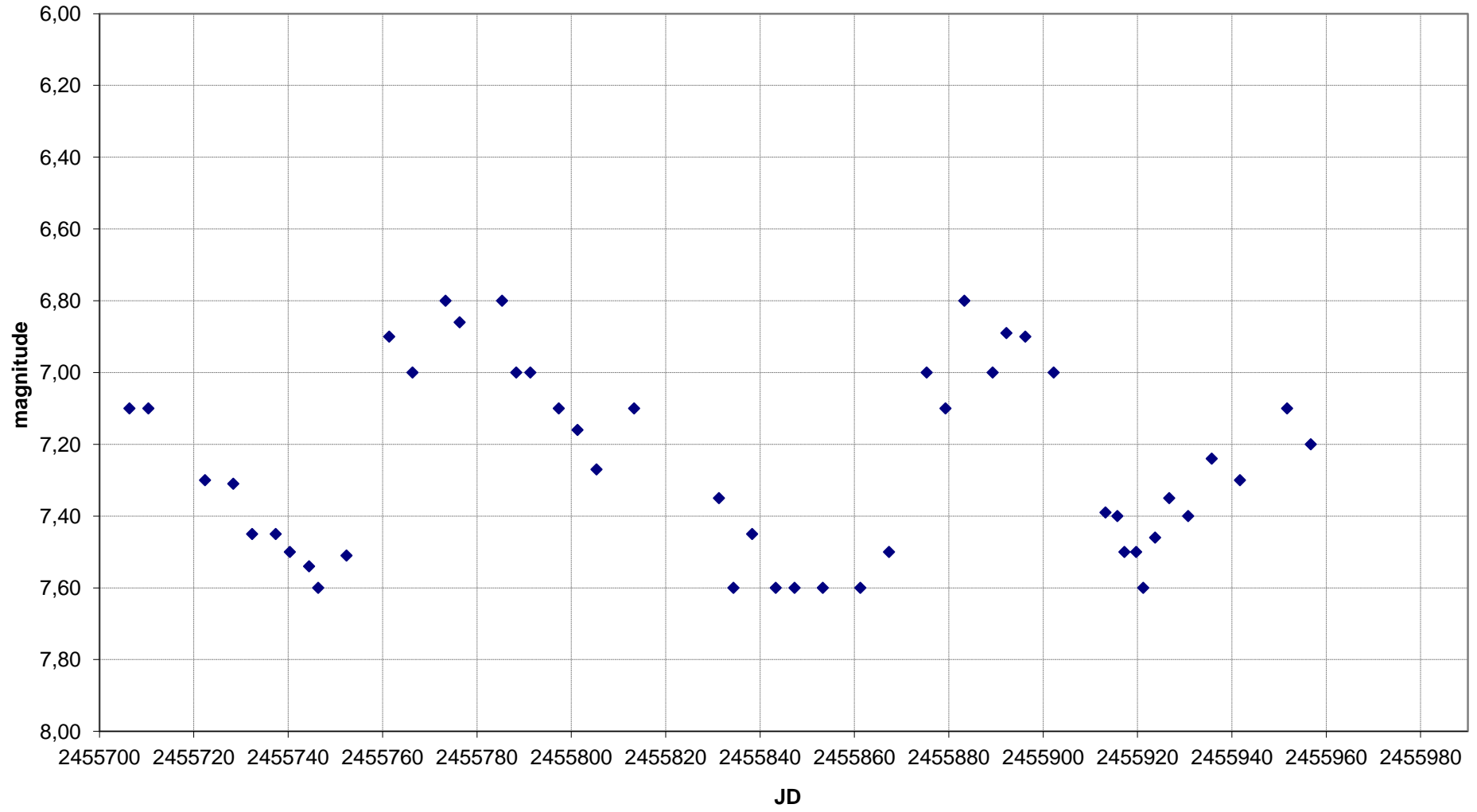
AF Cyg - Grafico al 30/01/2012
