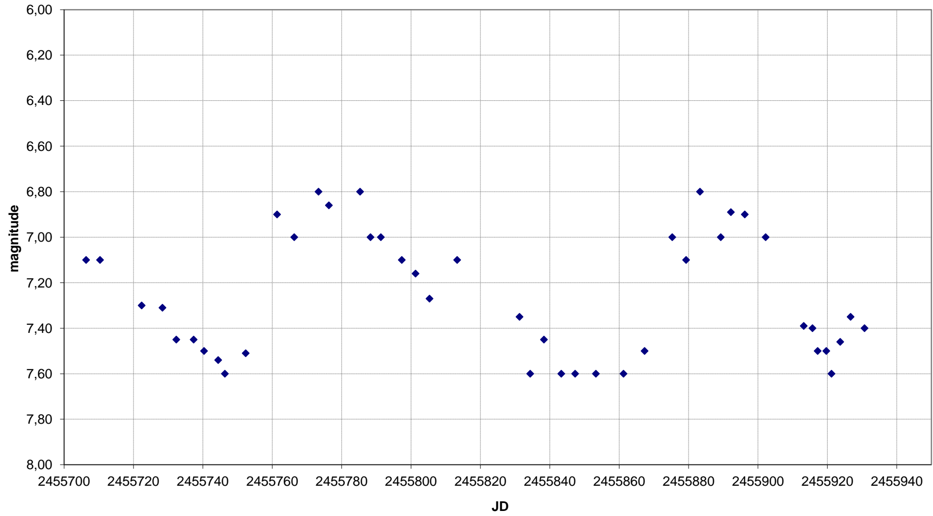
AF Cyg - Grafico al 04/01/2012
