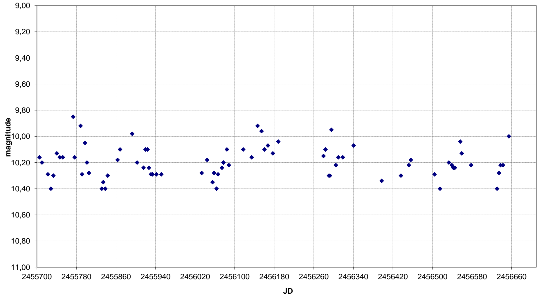
T CrB - Grafico al 28/12/2013
