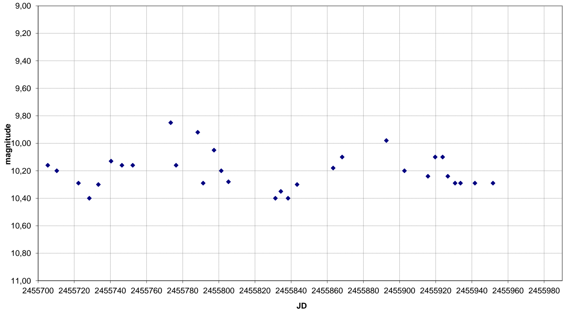
T CrB - Grafico al 25/01/2012
