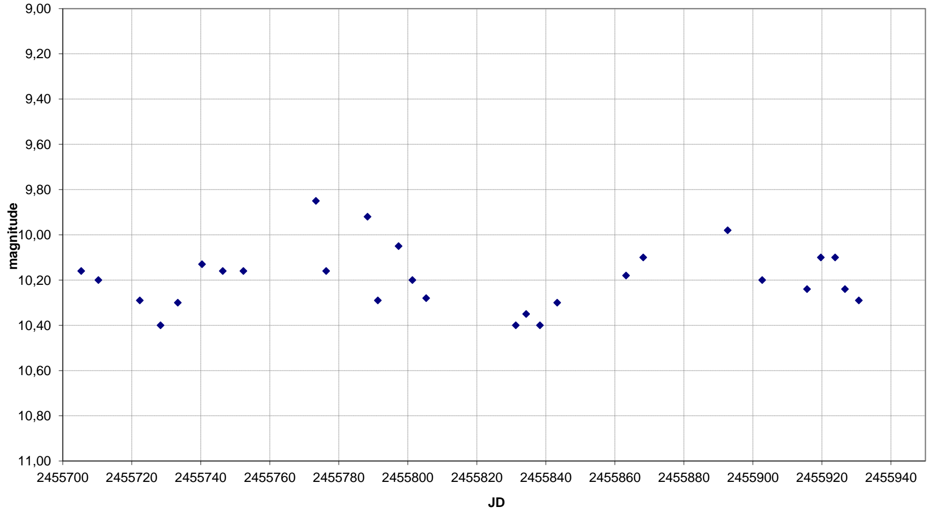
T CrB - Grafico al 04/01/2012
