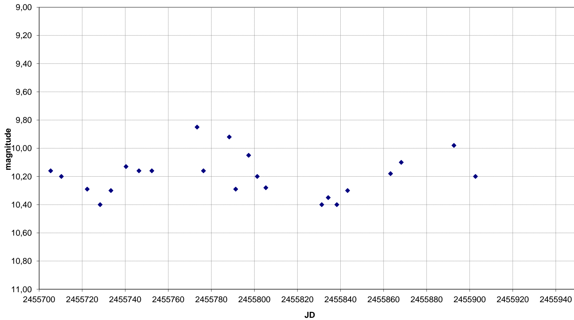
T CrB - Grafico al 07/12/2011
