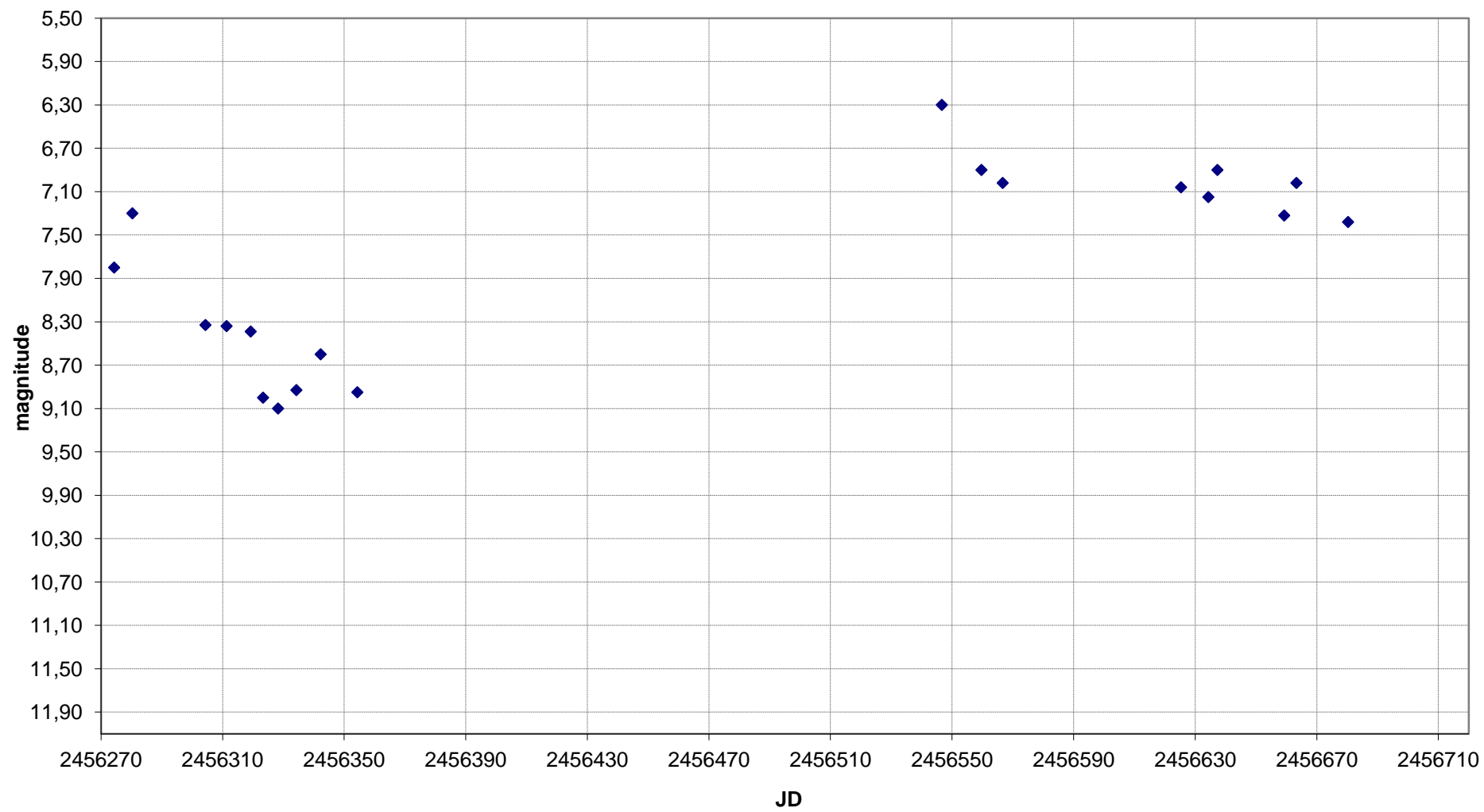
R Lep - Grafico al 22/01/2014
