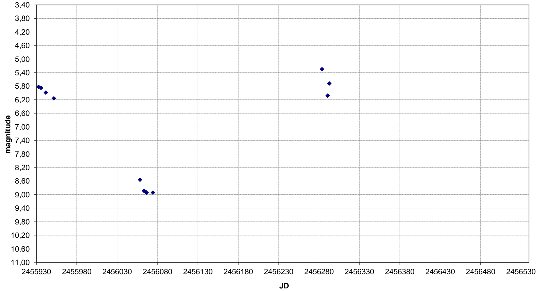
R Hya - Grafico al 31/12/2012
