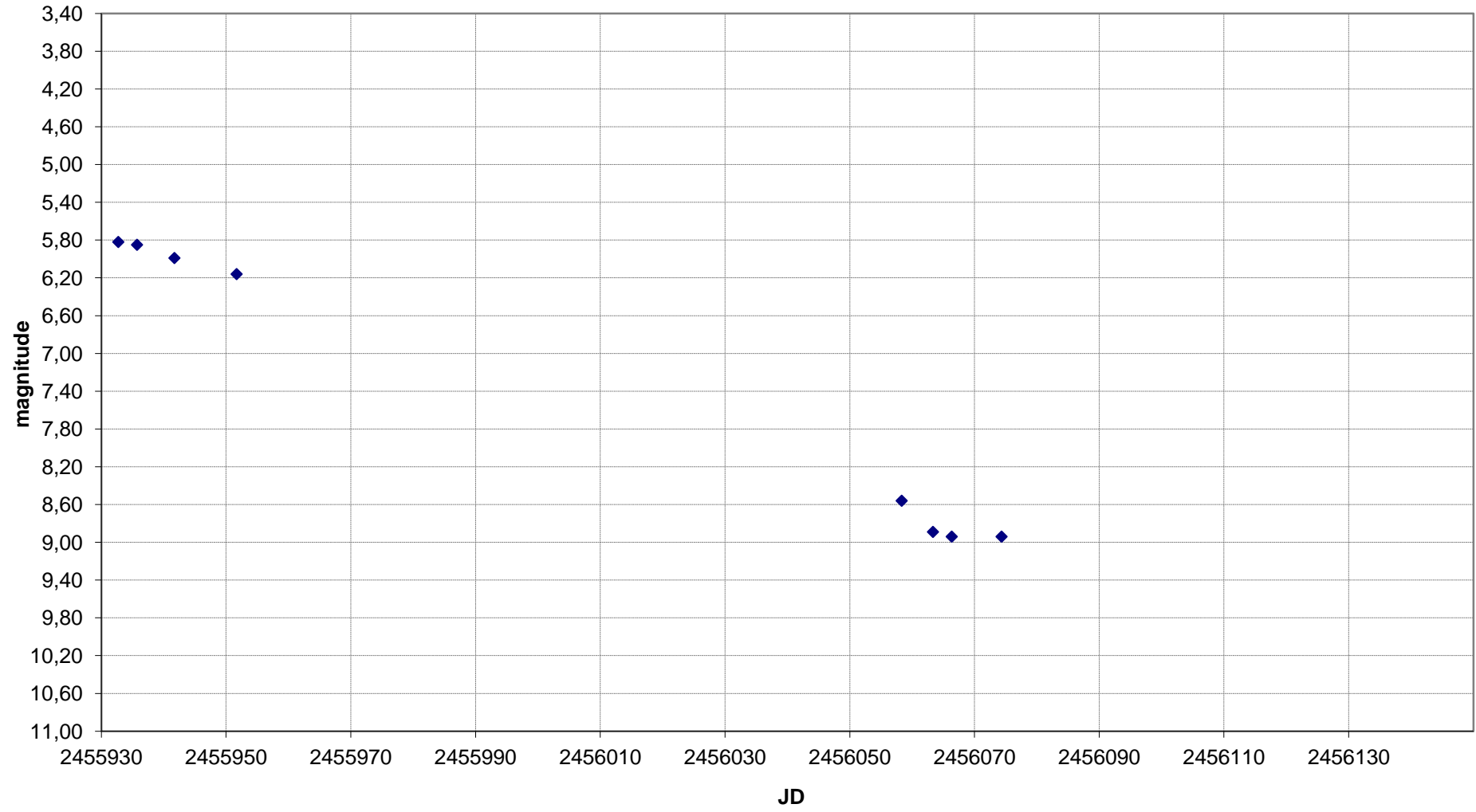
R Hya - Grafico al 26/05/2012
