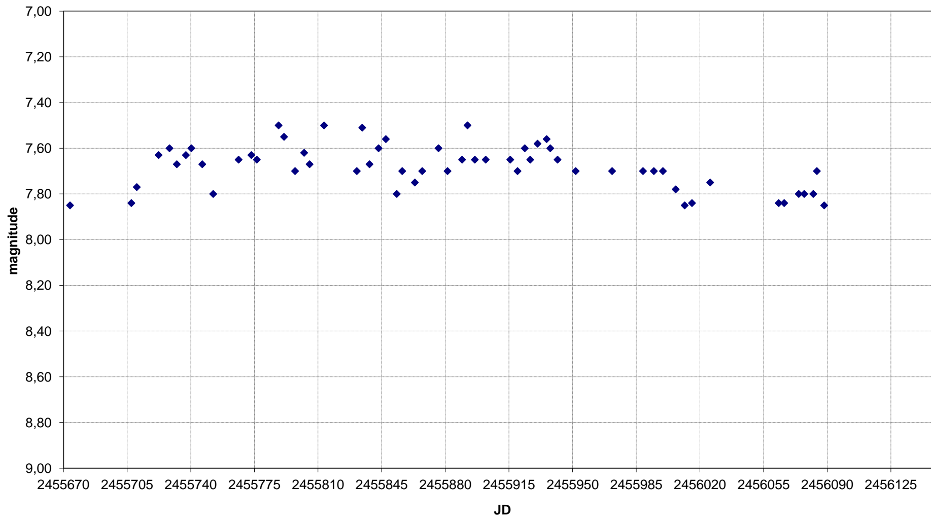
HK Lyr - Grafico al 09/06/2012
