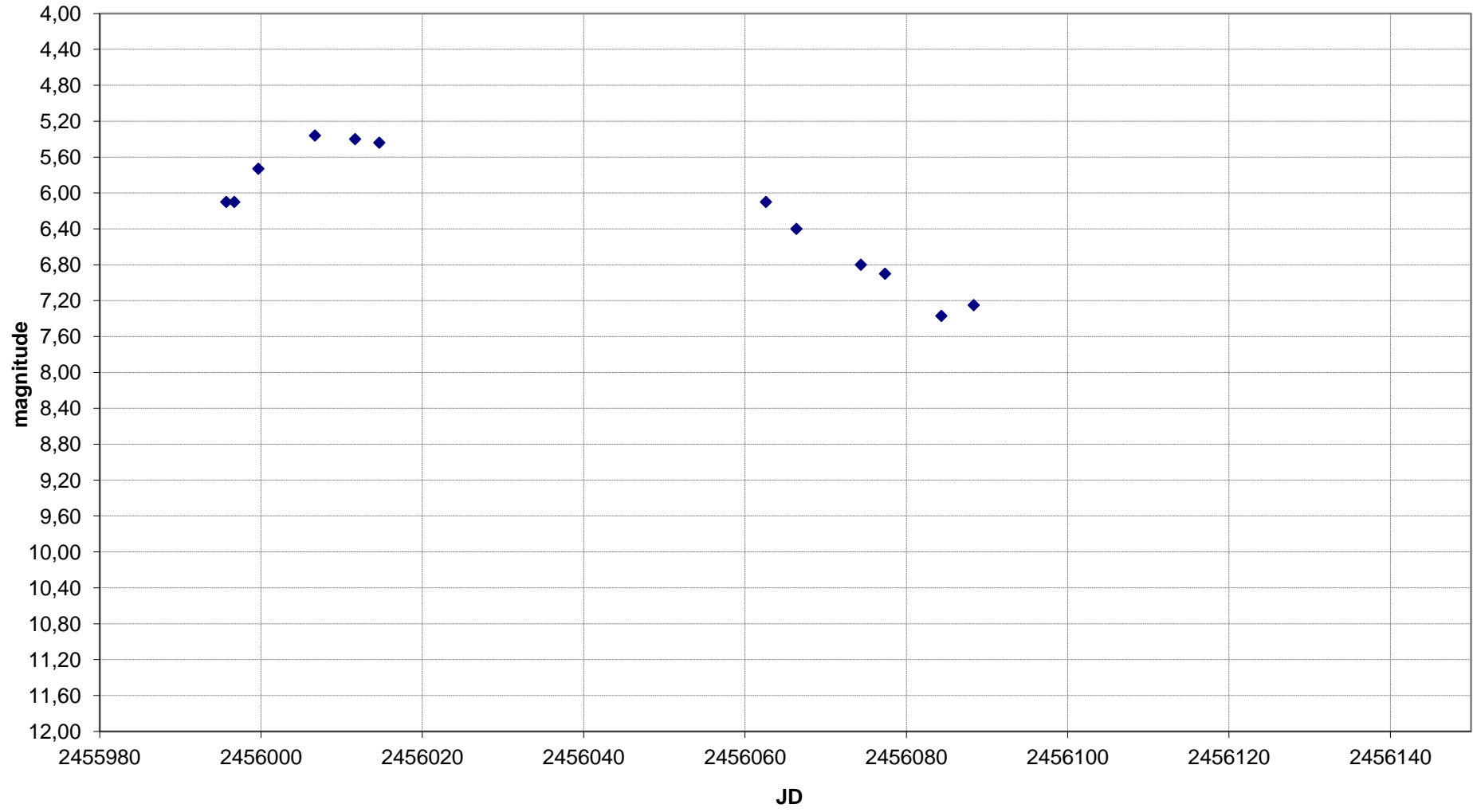
Chi Cyg - Grafico al 09/06/2012
