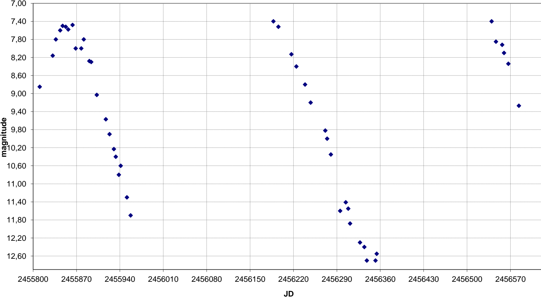
S CMi - Grafico al 18/10/2013
