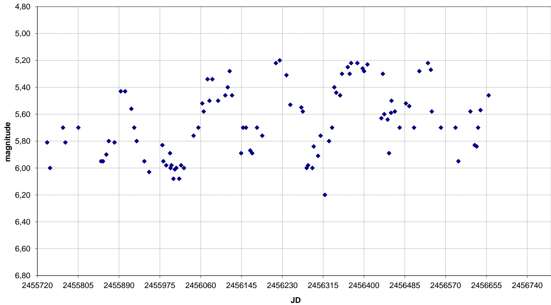
Y CVn - Grafico al 02/01/2014
