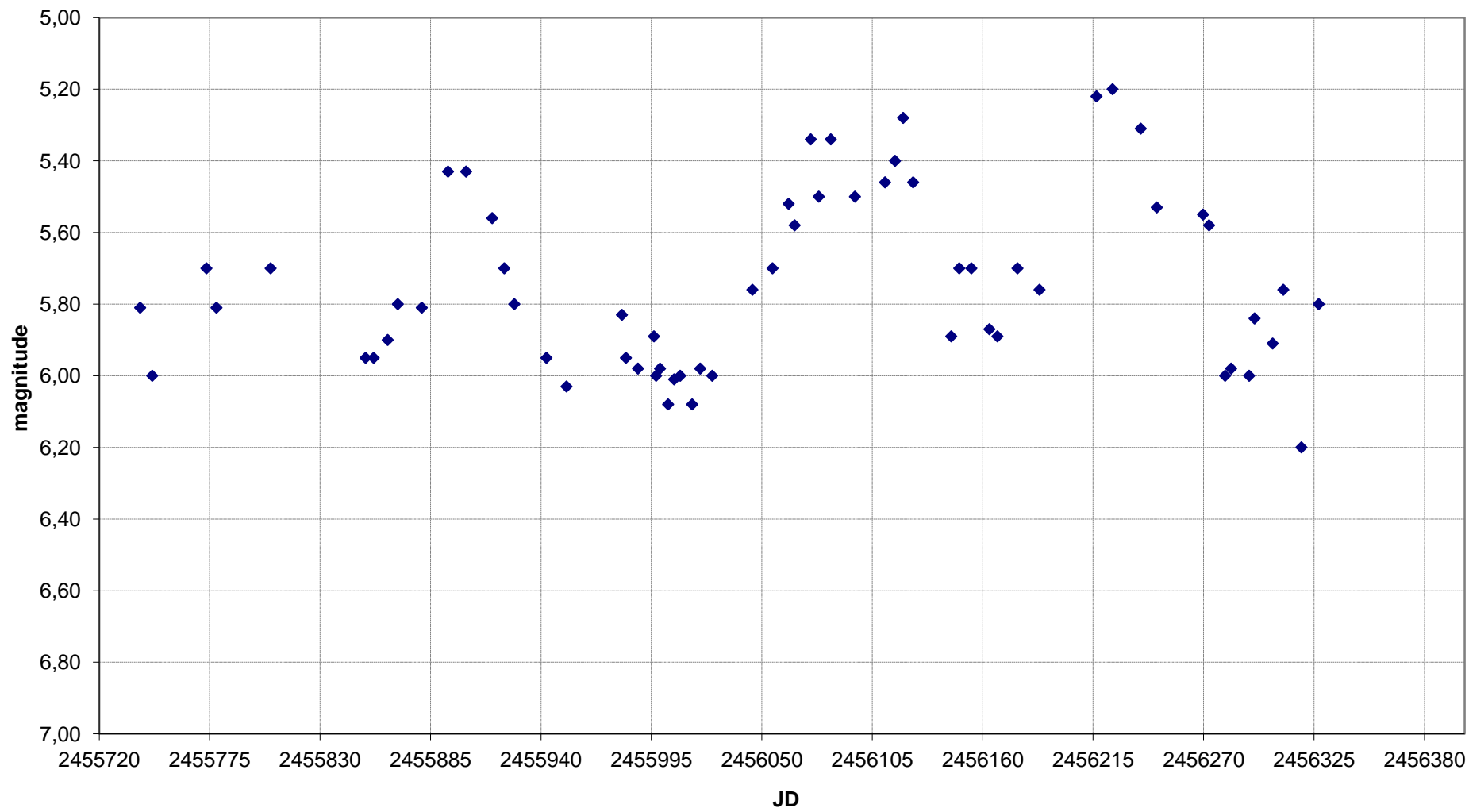
Y CVn - Grafico al 03/02/2013
