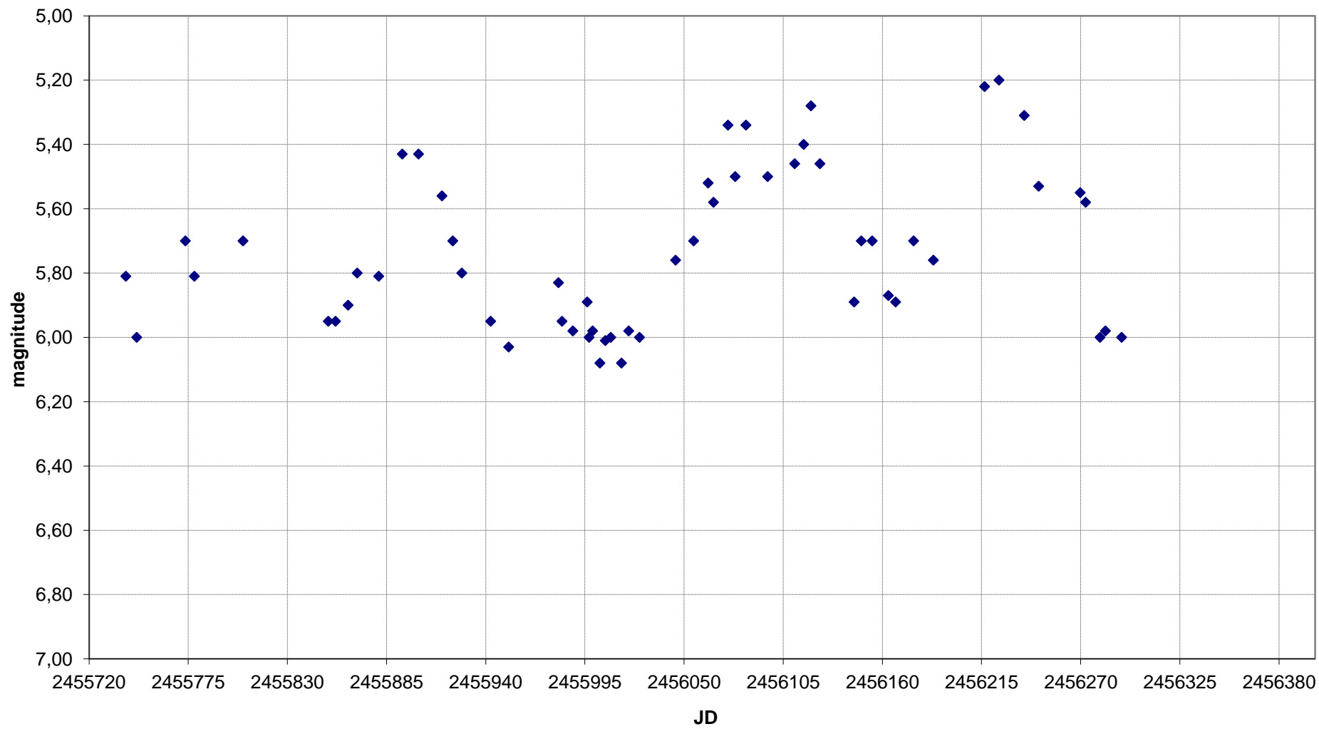
Y CVn - Grafico al 31/12/2012
